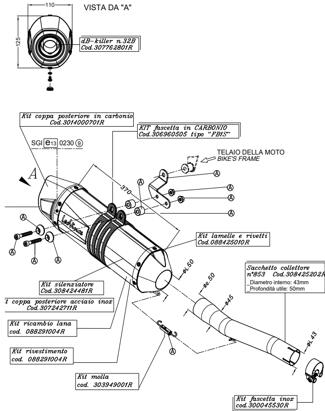
ART. 8424E SPARE PARTS
