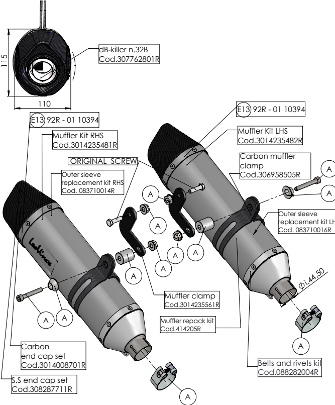
ART. 14235E SPARE PARTS
